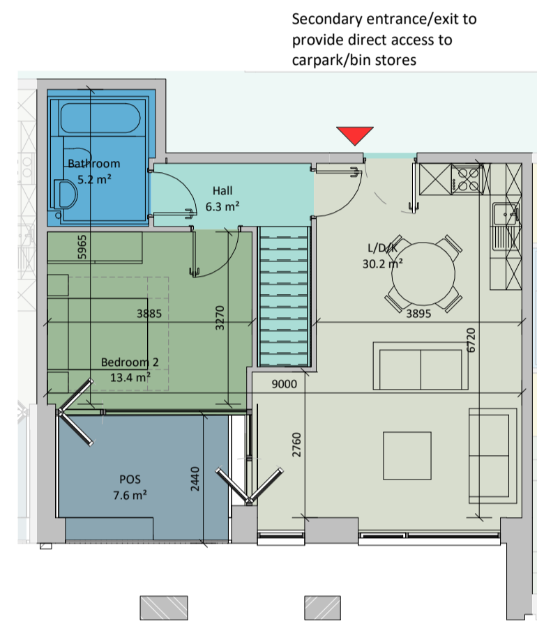
④ AT-2D1 - Upper Level 1:100
