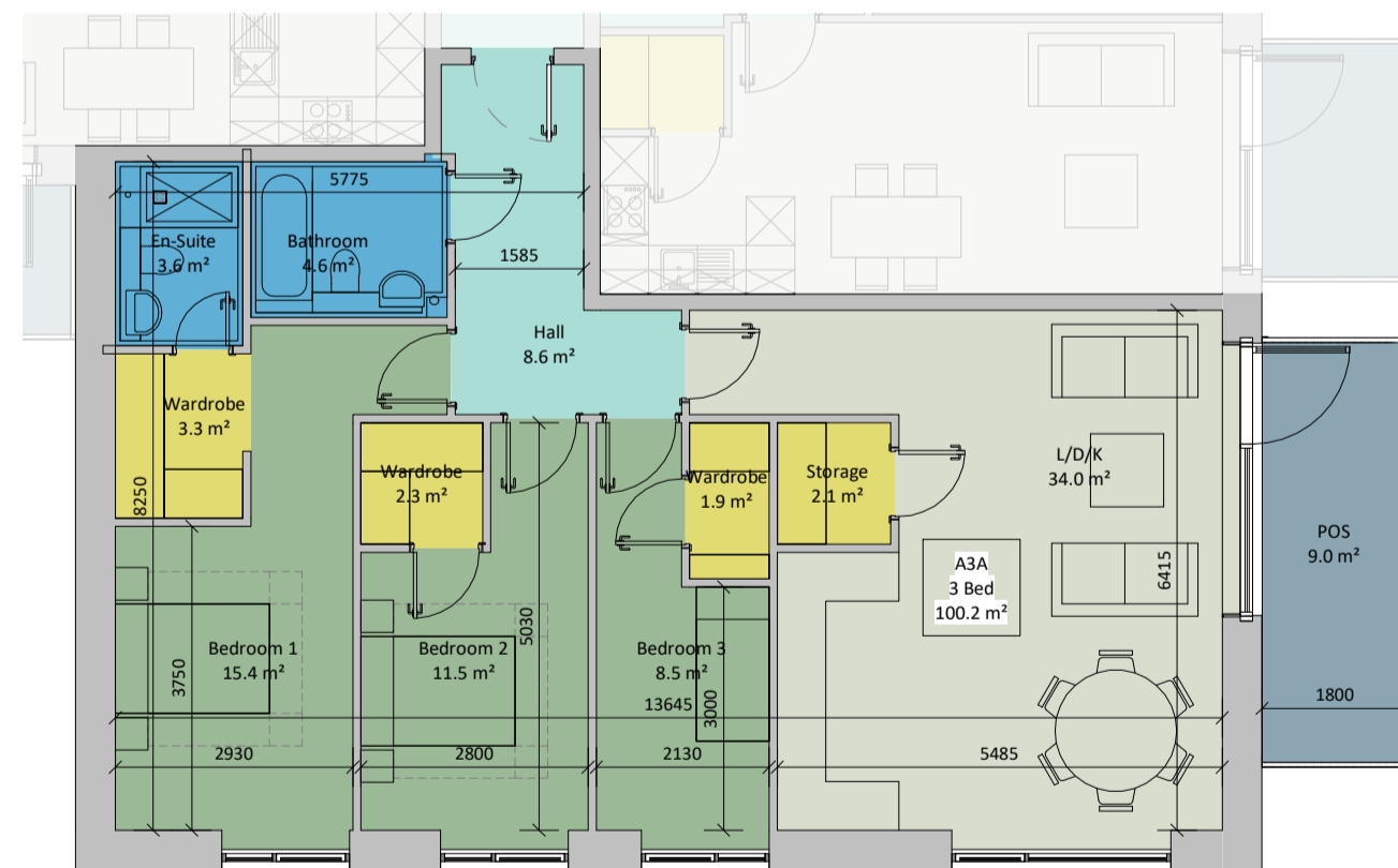
⑦ AT-A3A 1:100
